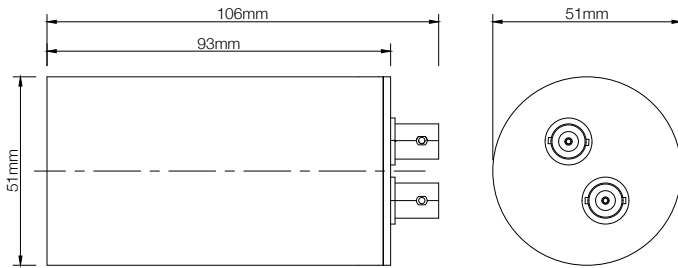
单位: mm 1.5英寸探测器
