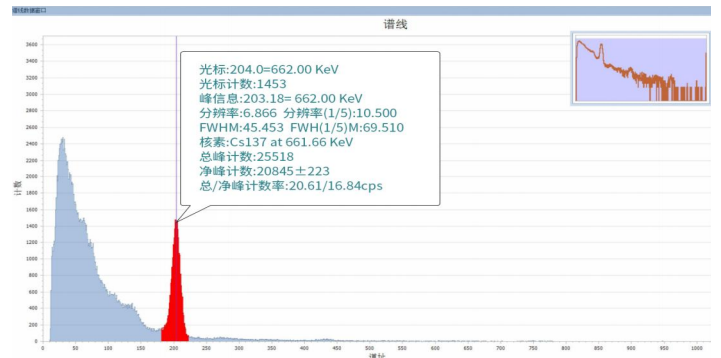
● 能谱测试: 能量分辨率 6.87% @662KeV
